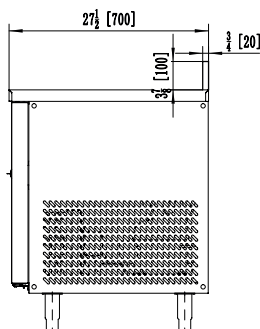
VISTA LATERAL
